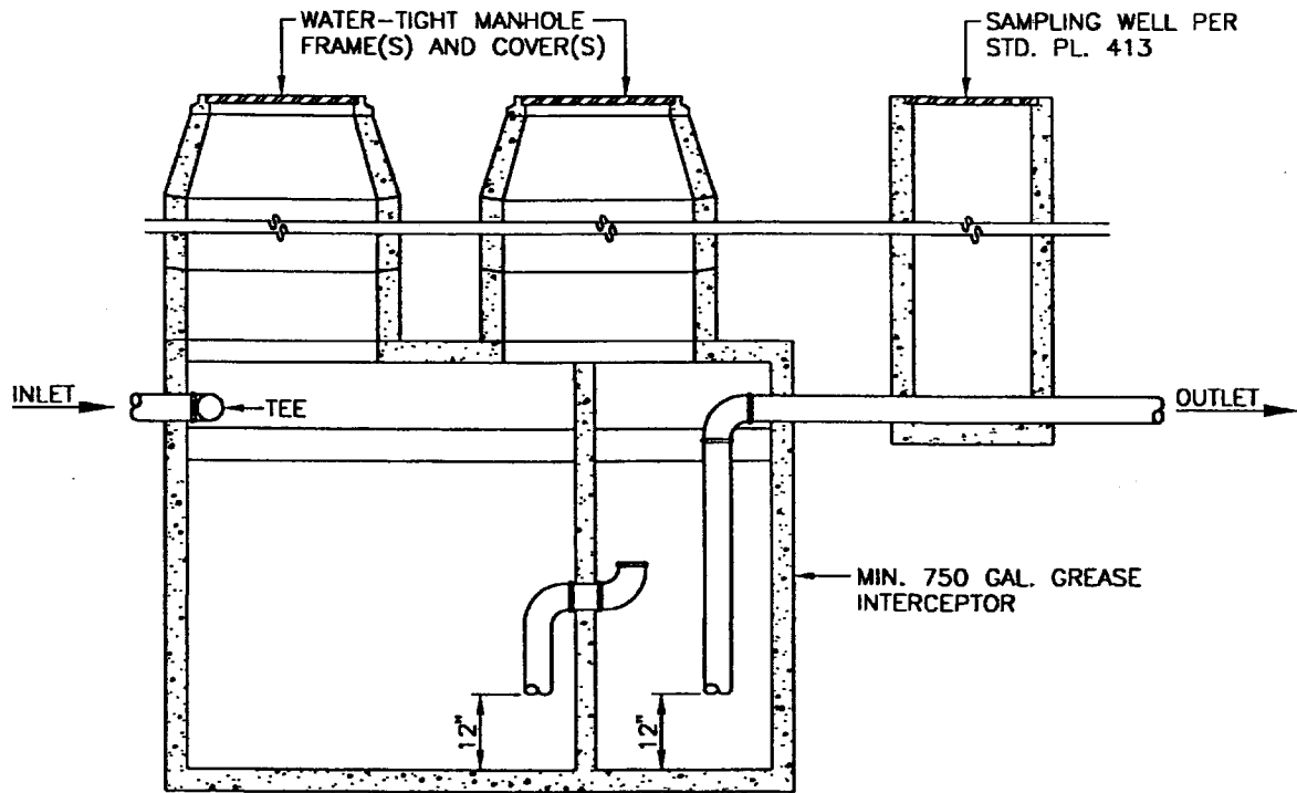
LONGITUDINAL SECTION
