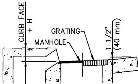
SECTION D-D
