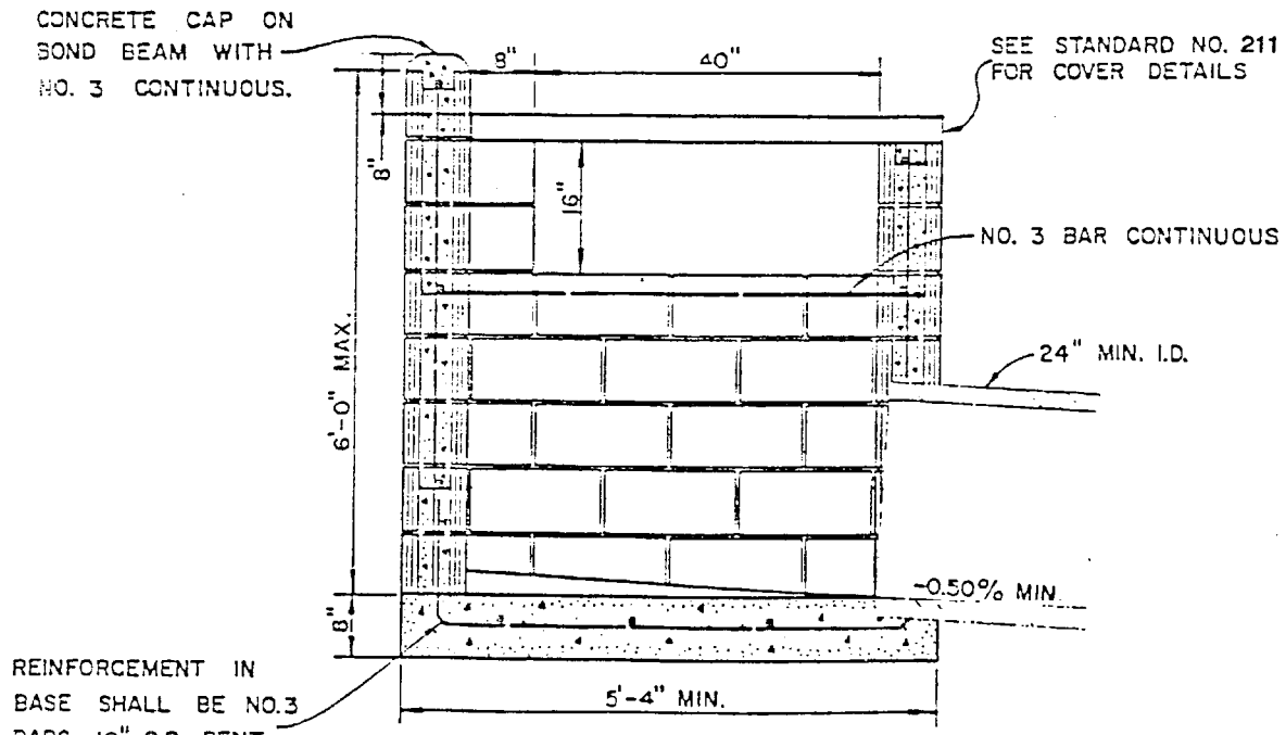
SECTION A-A
