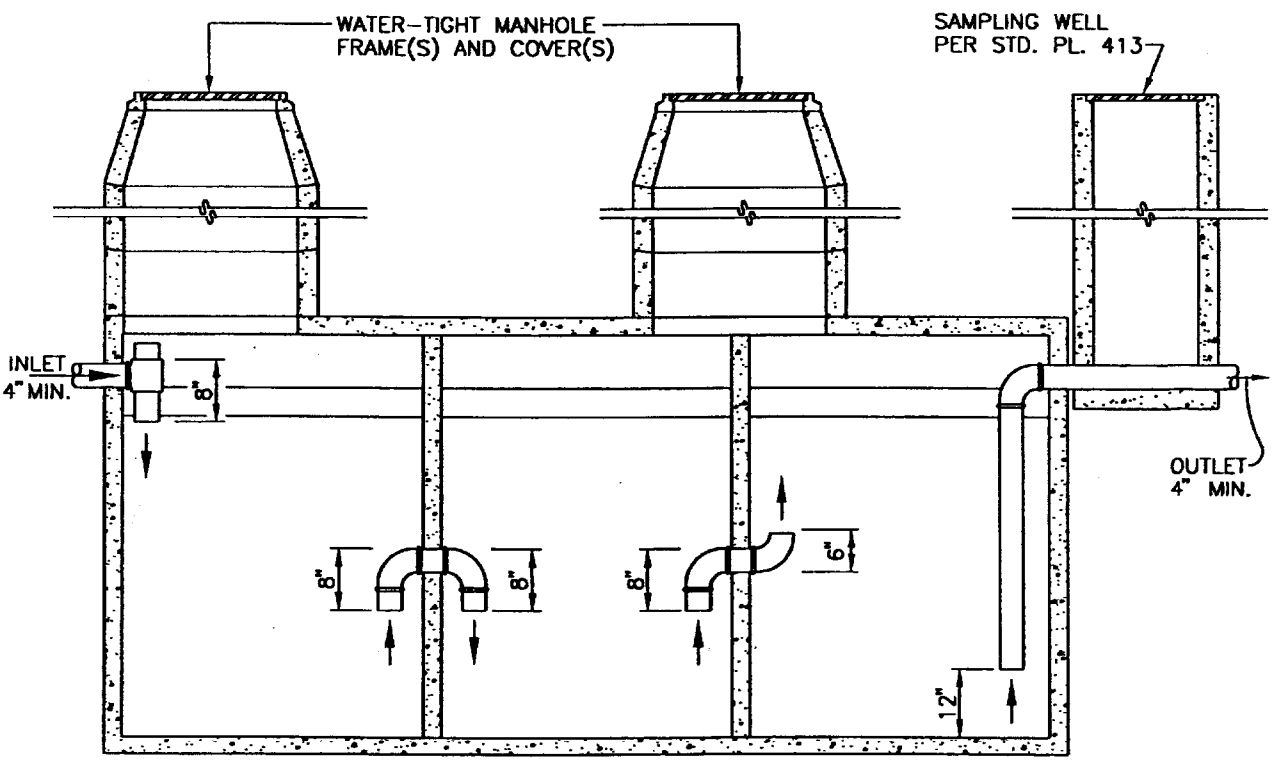
LONGITUDINAL SECTION
