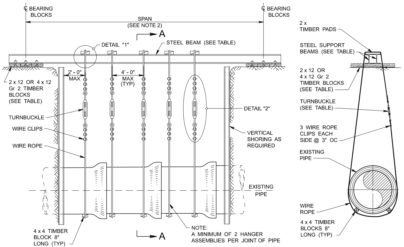
ELEVATION
