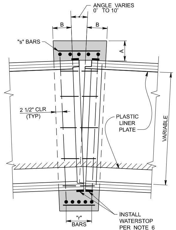
LONGITUDINAL SECTION
