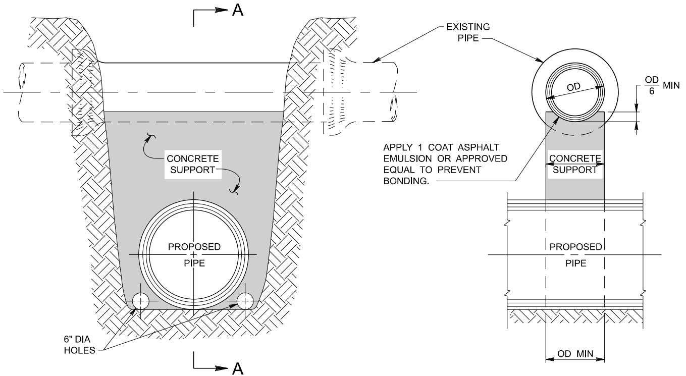
ELEVATION
