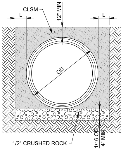
CLSM ENCASEMENT LOAD FACTOR = 2.8)
