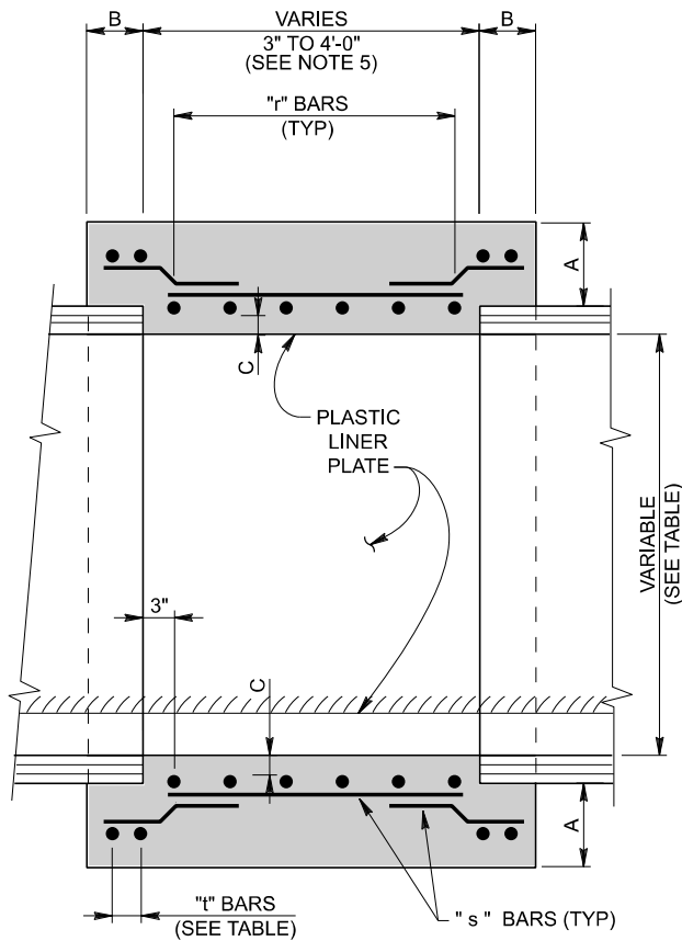
LONGITUDINAL SECTION
