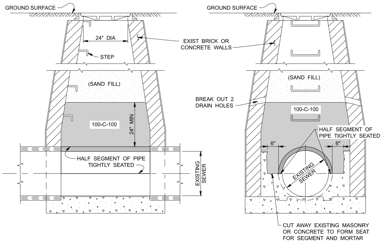
LONGITUDINAL SECTION
