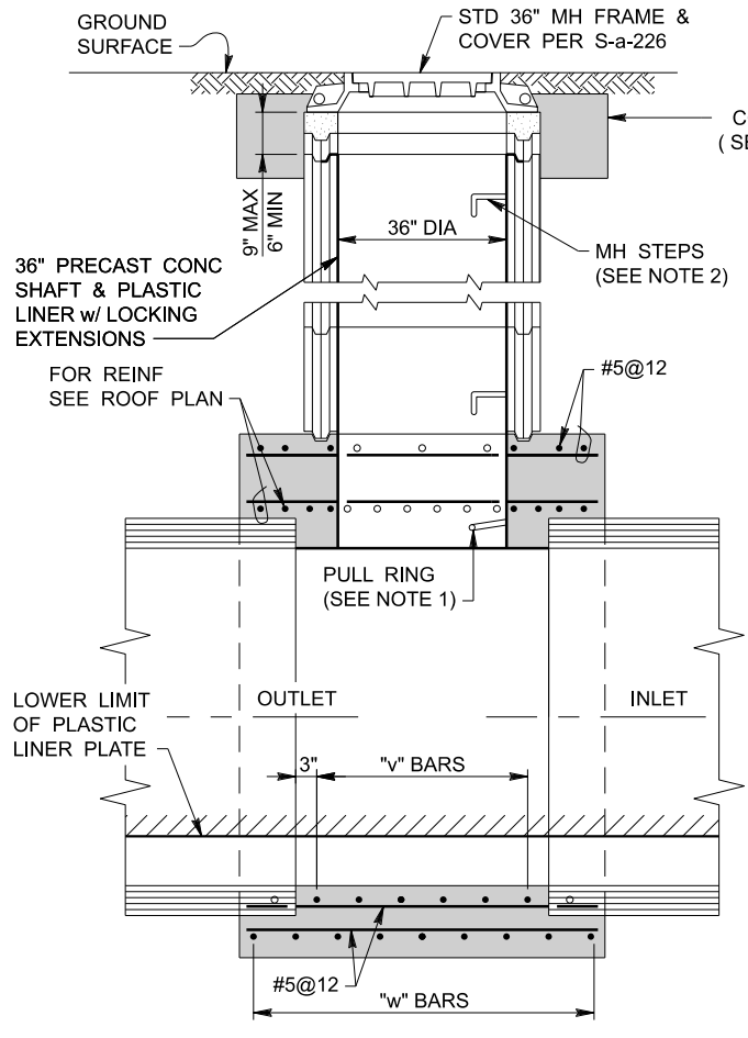
LONGITUDINAL SECTION
