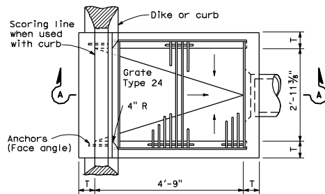
TYPE GDO
