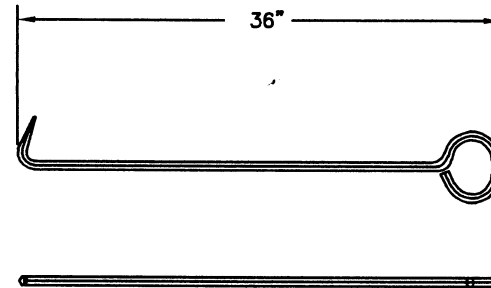
PULHEXANG36
