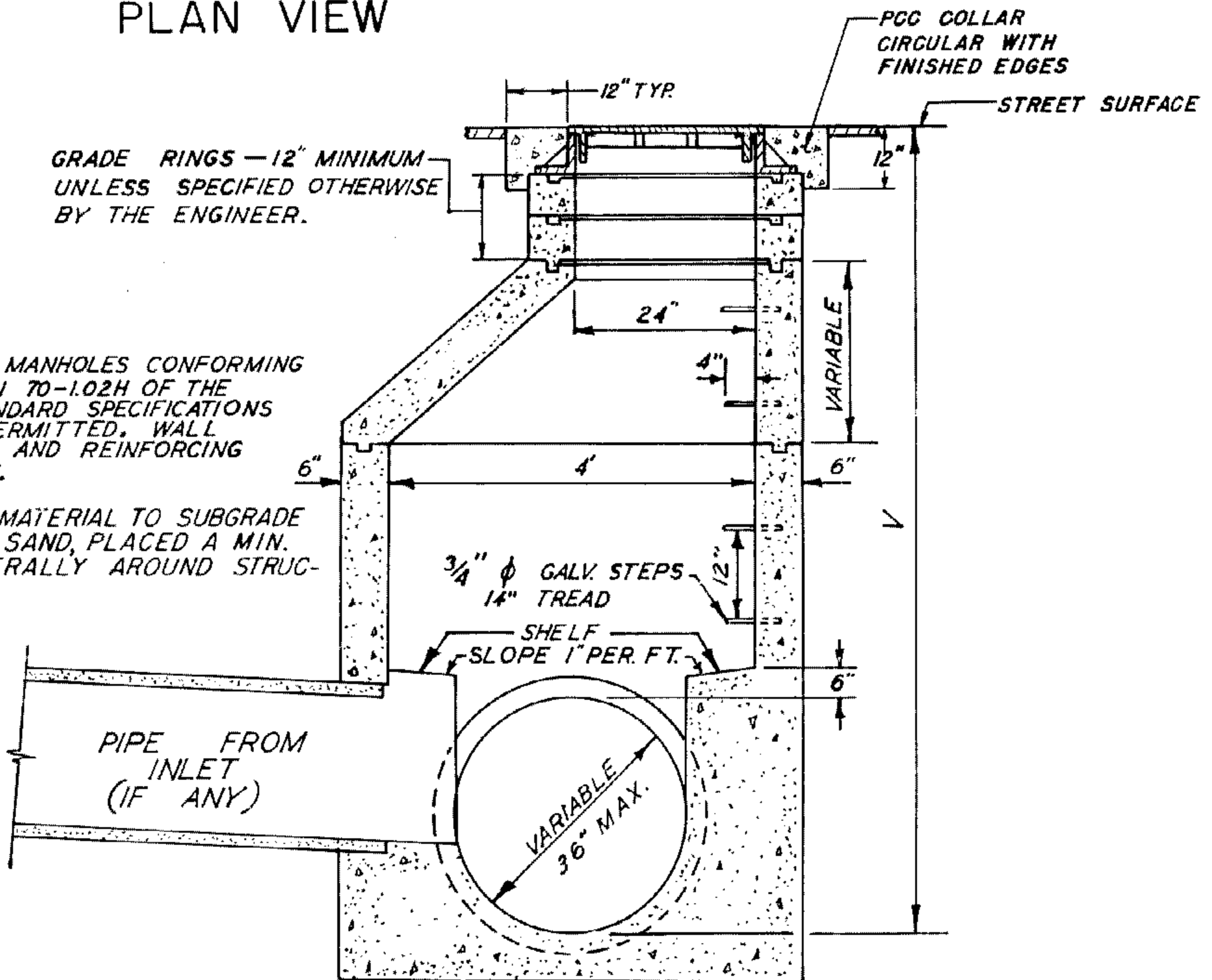
SECTION A-A
